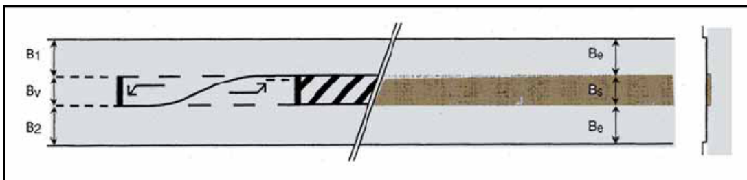
Soluzione con superficie non transitabile interamente o parzialmente attraversabile dai pedoni e dai ciclisti
