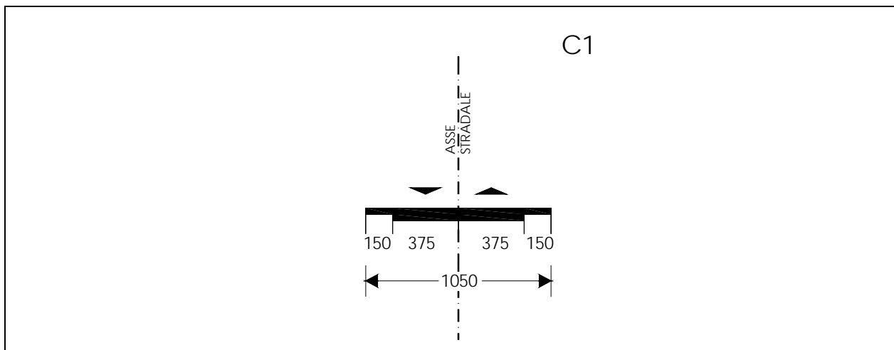
Fig. 1. 1 Strada extraurbana secondaria (Tipo C1): piattaforma stradale
