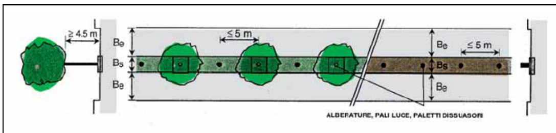
Soluzione con superficie non carrabile con presenza di essenze arboree o arbusti
